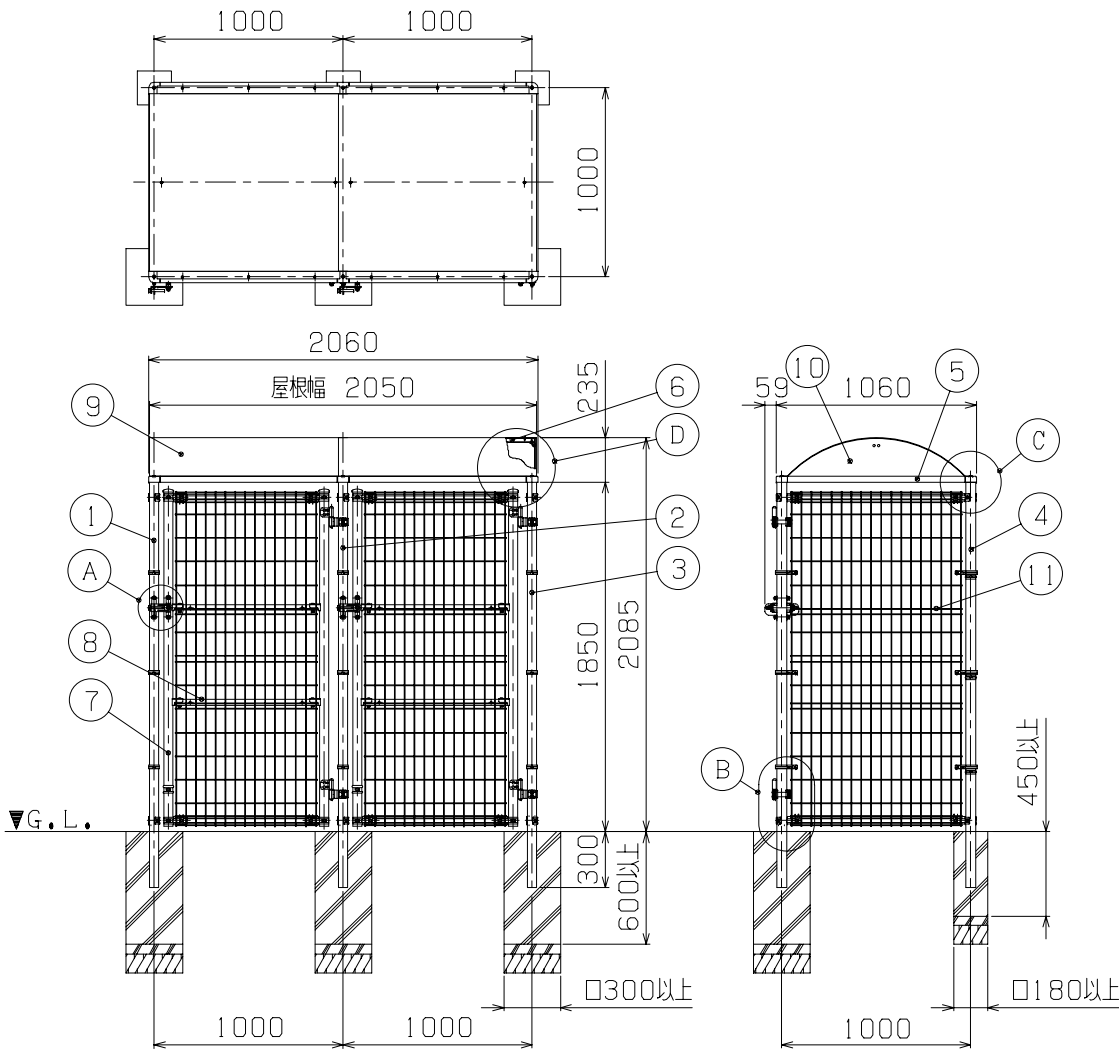
据付図 (1/40)
