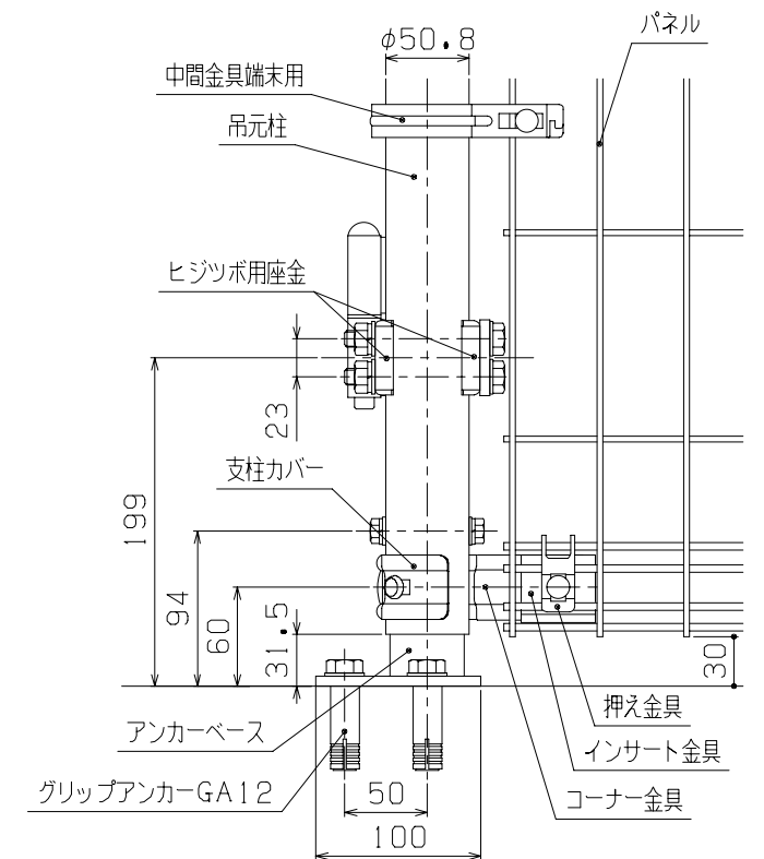
B部詳細図 (1/5)
