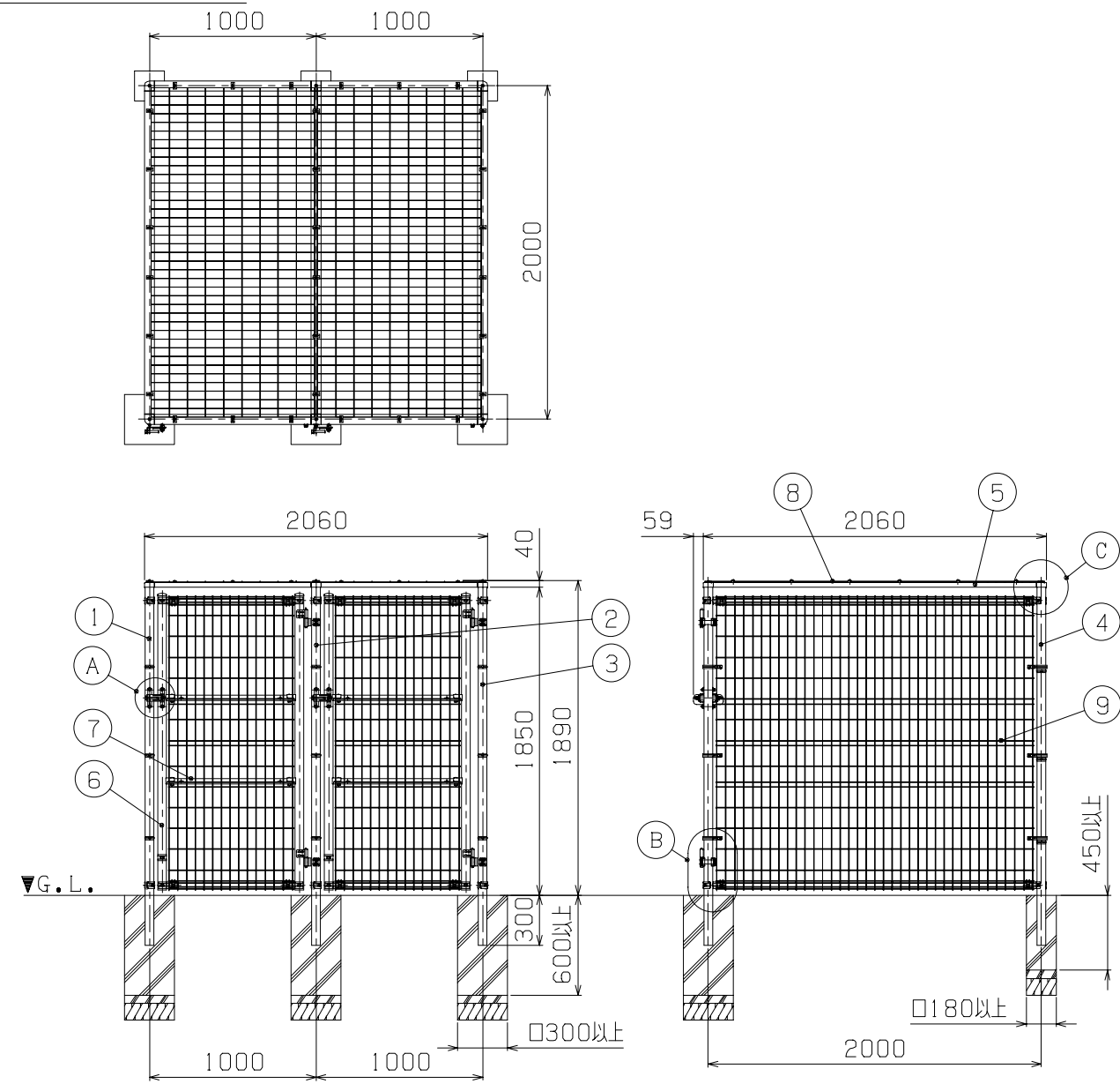
据 付 図 (1/40)
