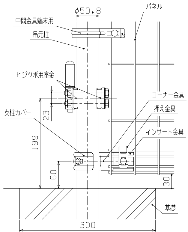
B 部 詳 細 図 (1/5)
