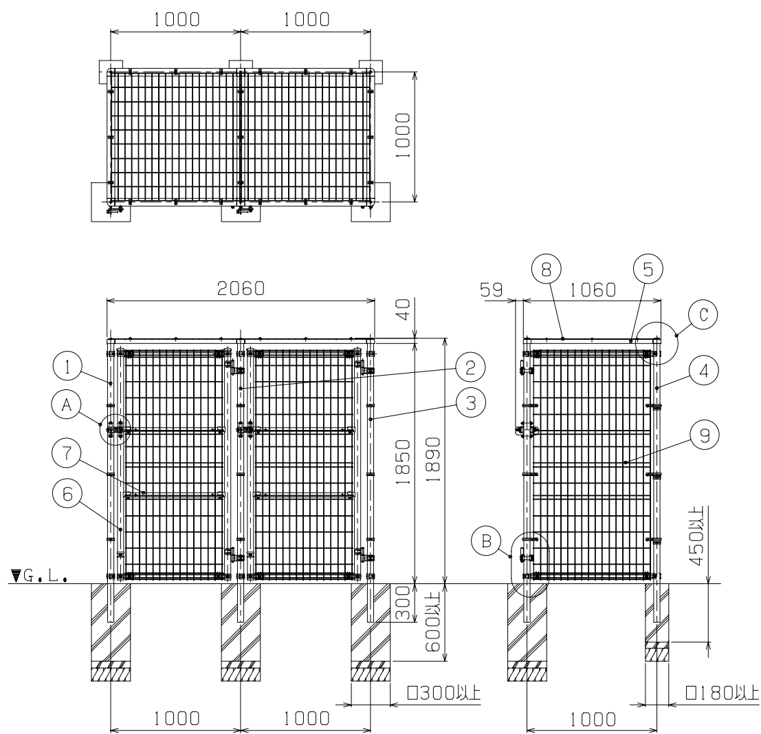
据付図 (1/40)
