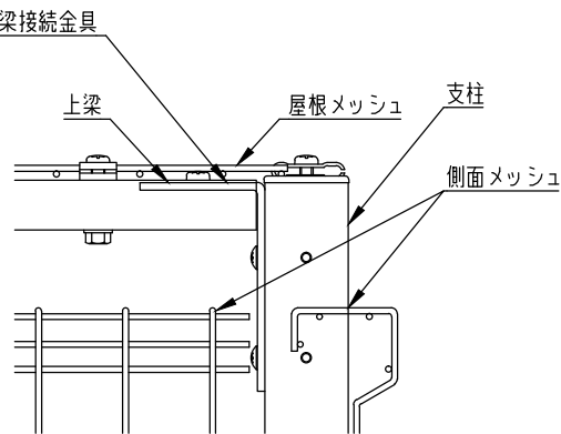
B 部 詳 細 図 (S = 1 / 5)
