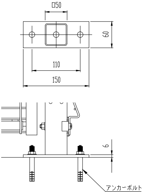
C 部 詳 細 図 (S = 1 / 5)
