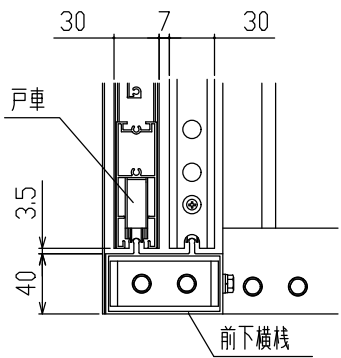
A部断面図 (S = 1 / 5)
