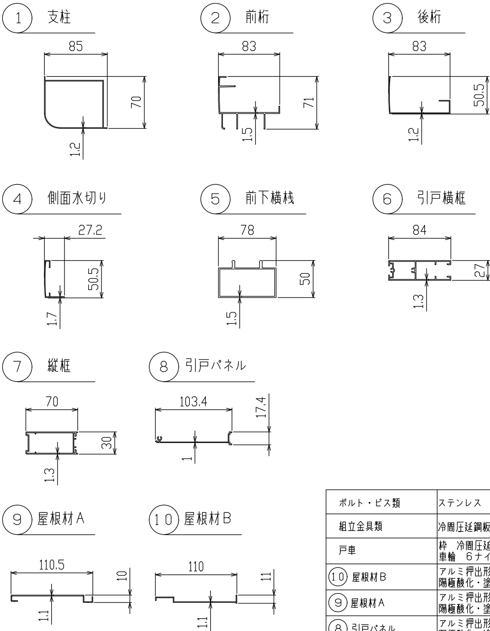
主要部材断面図 (S = 1 / 5)
