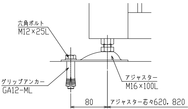
B部詳細図 (S = 1 / 5)
