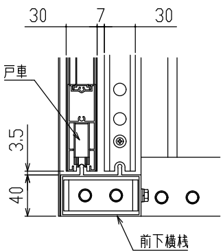
A部断面図 (S = 1 / 5)
