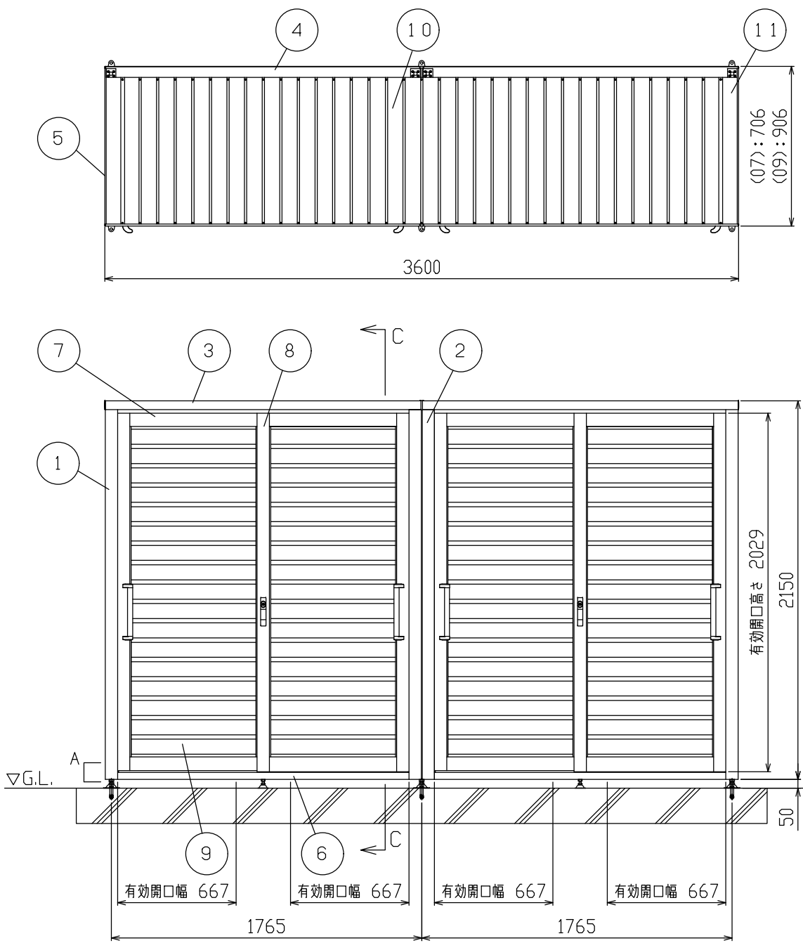
据付図（S＝1／30）
