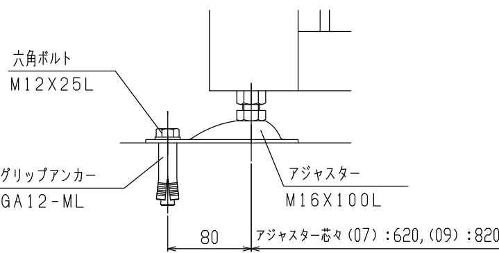
B部詳細図（S＝1／5）
