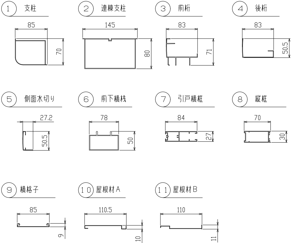
主要部材断面図（S＝1／5）
