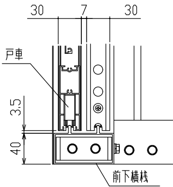
A部におけるC-C線断面図（S＝1／5）
