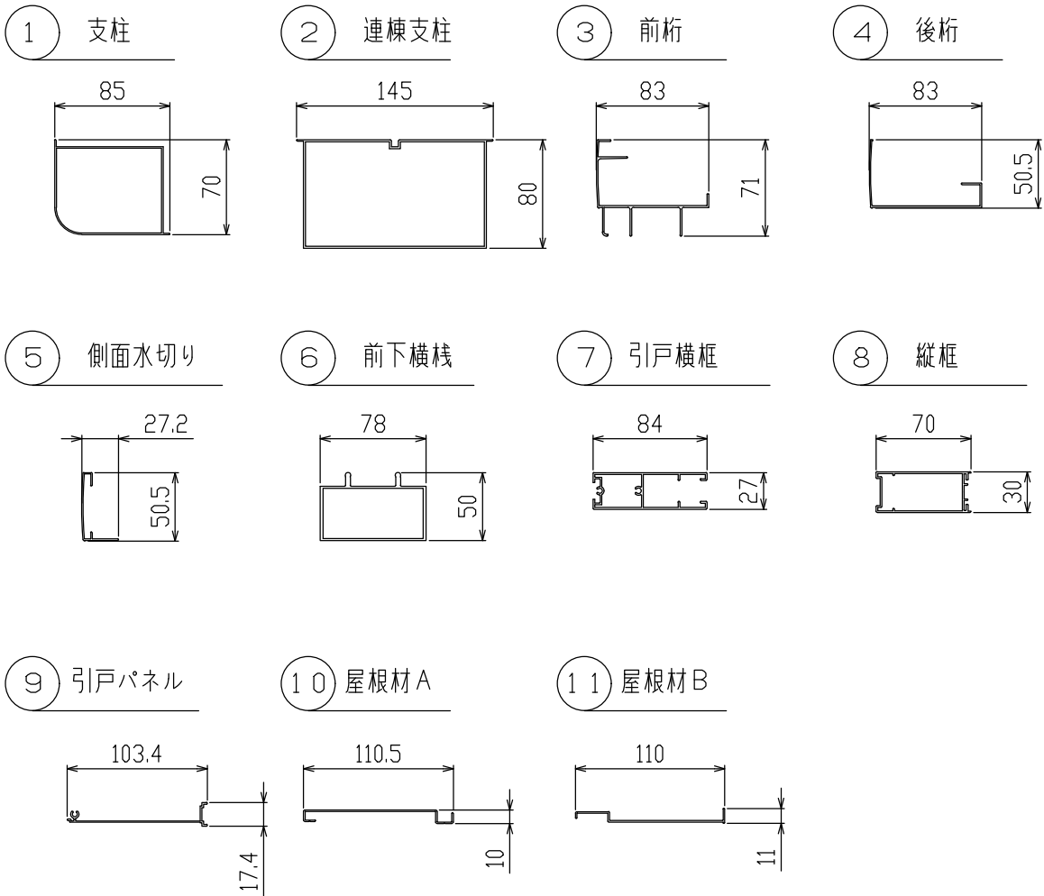
主要部材断面図（S＝1／5）
