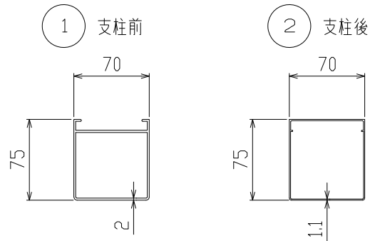
主要部材断面図 (S=1/5)
