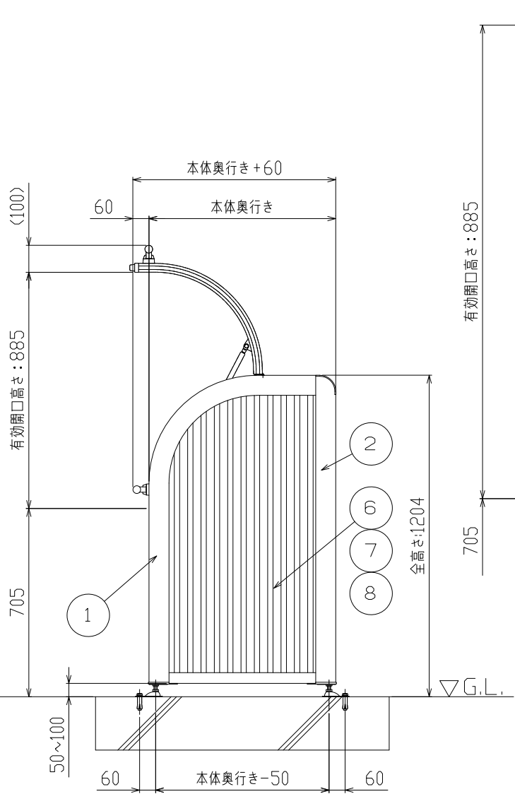
主要部材断面図 (S=1/5)
