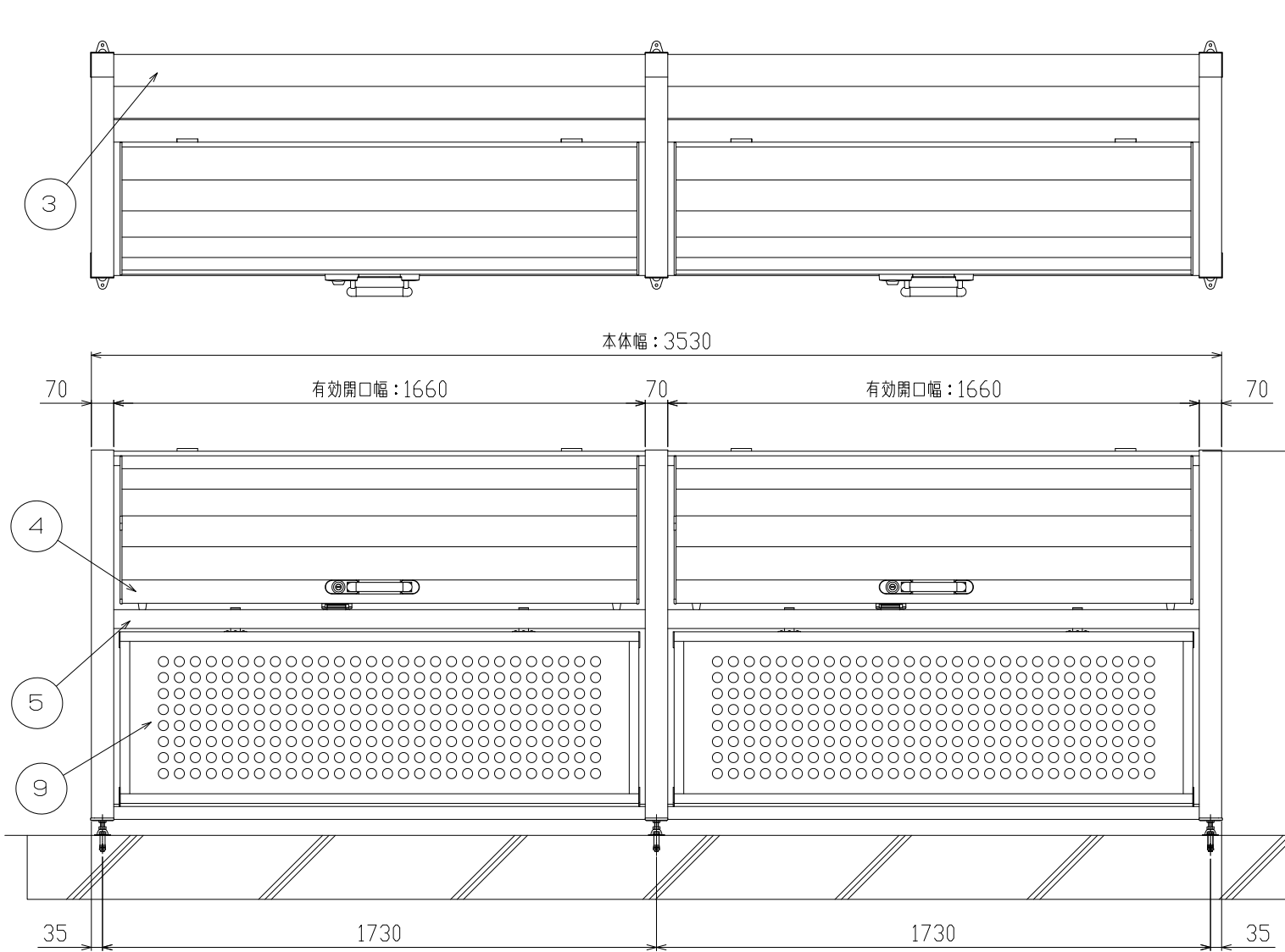
据付図 (S=1/20)
