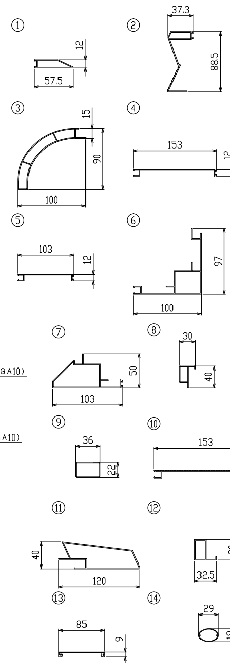
主要部材断面 (S=1/5)
