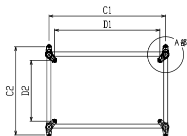
アンカー設置図 (S=1/20)
