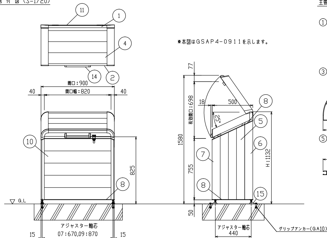
アンカー設置図 (S=1/20)
