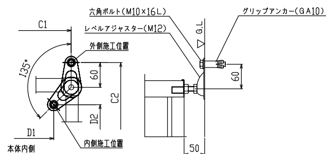
A部詳細図 (S=1/5)
