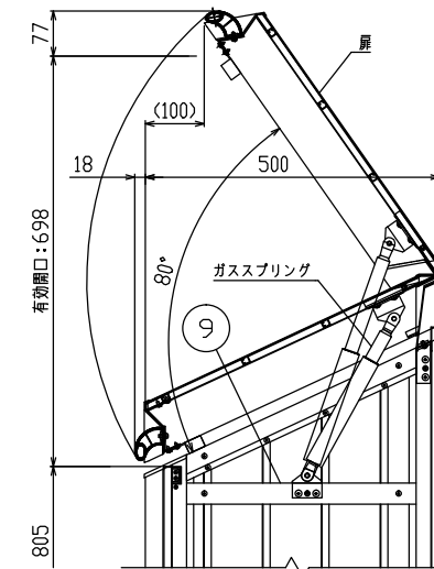
扉・ガススプリング納り詳細図 (S=1/10)
