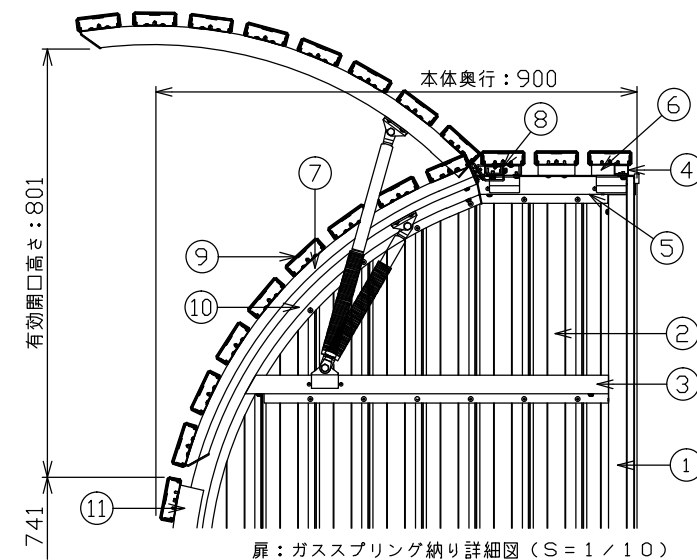
扉：ガススプリング納り詳細図 (S=1/10)
