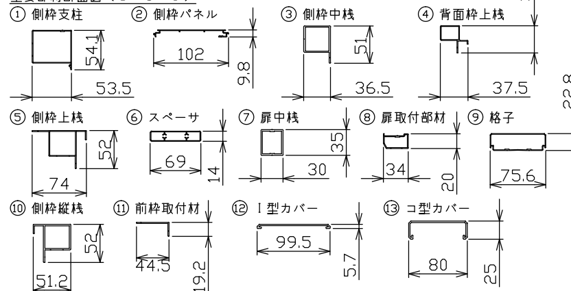
主要部材断面図 (S=1/5)
