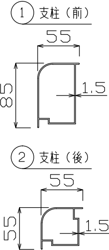
主要部材断面図 (S = 1 / 5)
