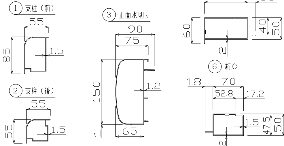
主要部材断面図 (S = 1 / 5)
