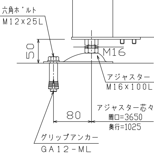
C部詳細図 (S = 1 / 5)
