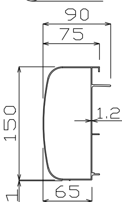
③ 正面水切り
