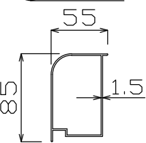
① 支柱 (前)
