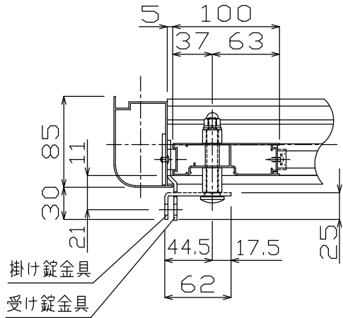
A - A断面図 (S = 1 / 5)
