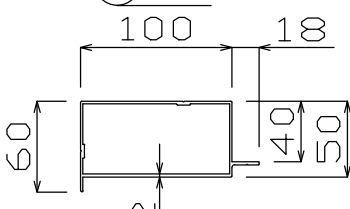
④ 桁 A
