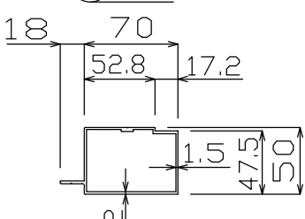
⑥ 桁 C
