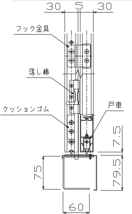
C - C断面図 (S = 1 / 5)
