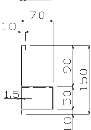
⑤ 桁 B
