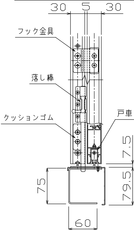
C - C断面図 (S = 1 / 5)
