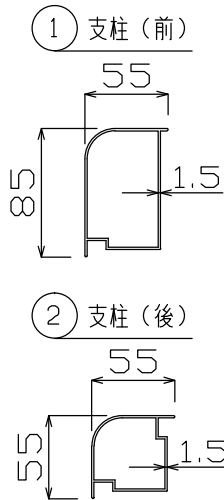
主要部材断面図 (S = 1 / 5)
