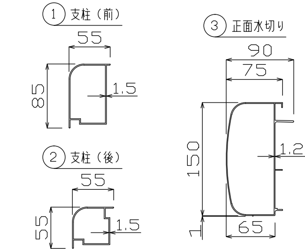
主要部材断面図 (S = 1 / 5)
