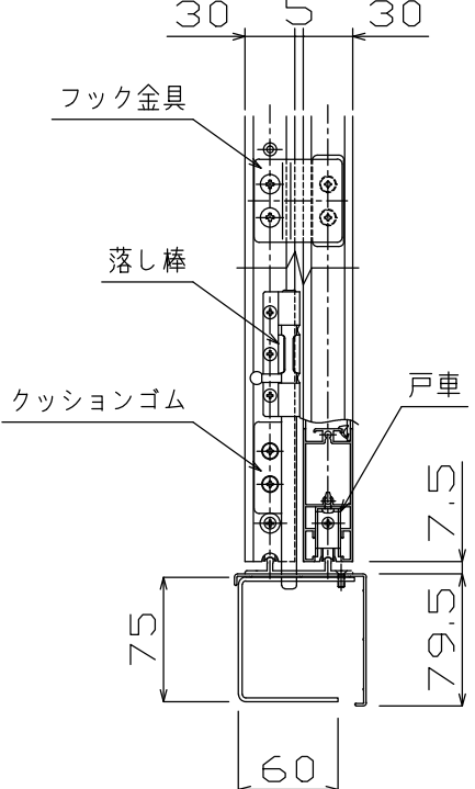
C - C断面図 (S = 1 / 5)
