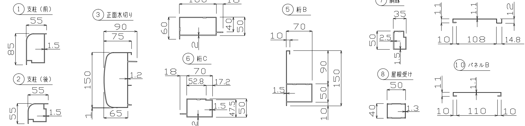
主要部材断面図 (S = 1 / 5)
