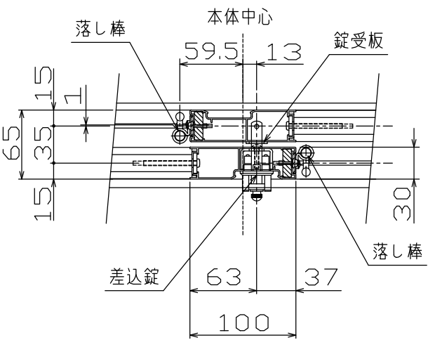
A - A断面図 (S = 1 / 5)
