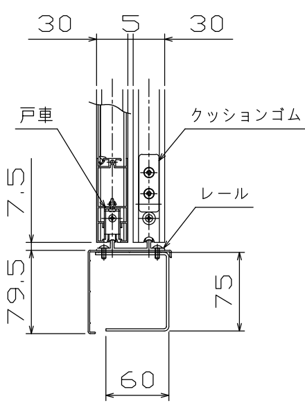
B - B断面図 (S = 1 / 5)
