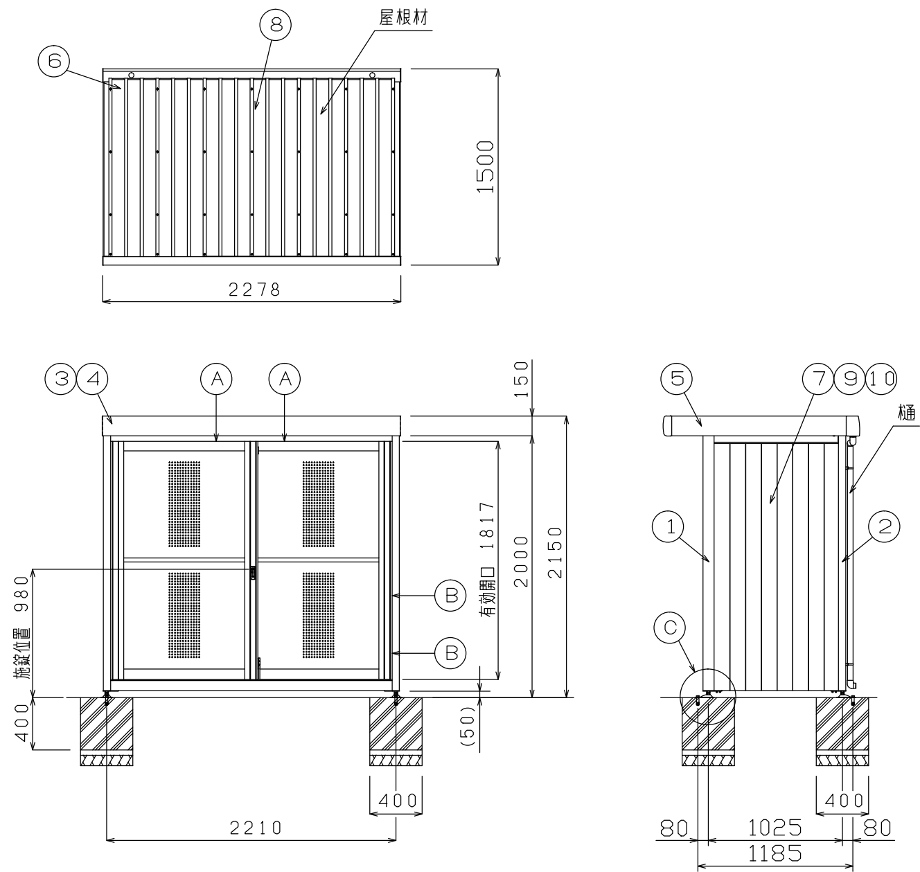
主要部材断面図 (S = 1 / 5)
