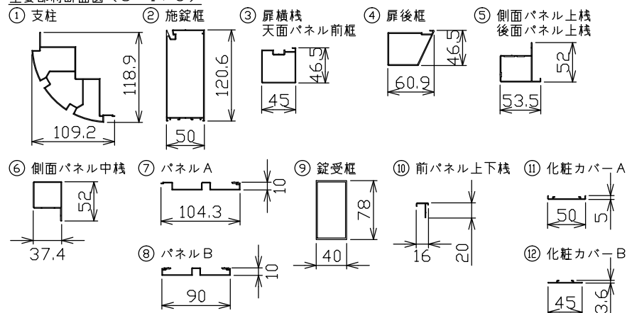
主要部材断面図 (S=1/5)
