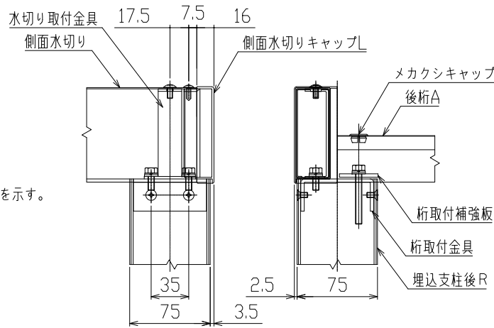
C部詳細図 (S=1/5)
