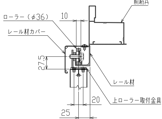
A-A詳細 (S=1/3)
