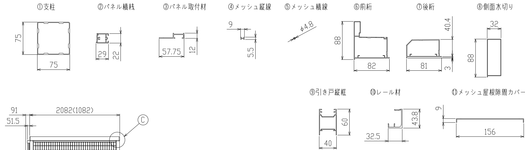
主要部材断面 (S=1/5)
