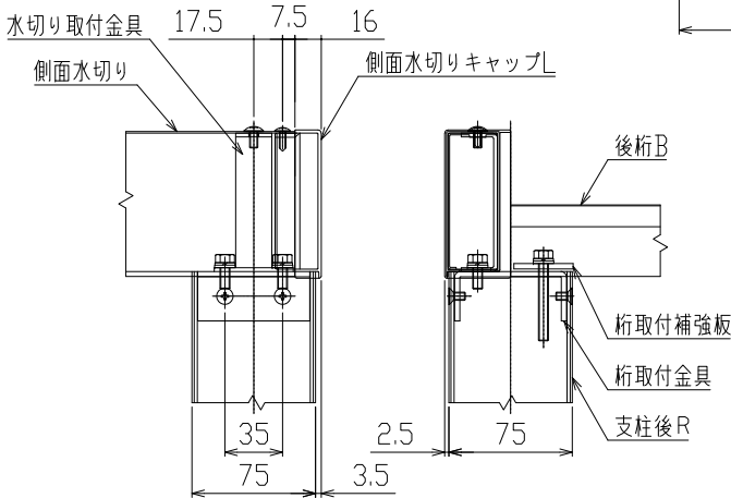
C部詳細図 (S=1/5)
