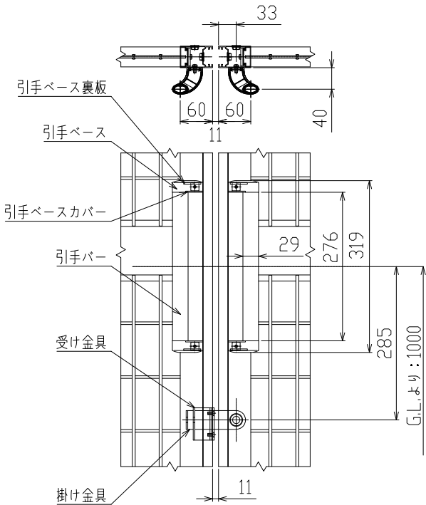
A部詳細図 (S=1/10)
