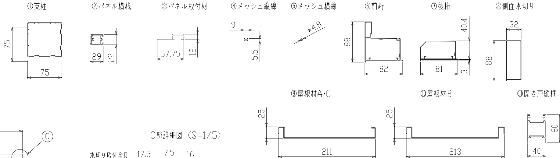
主要部材断面 (S=1/5)
