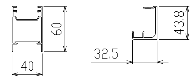
⑨引き戸縦框 ⑩レール材
