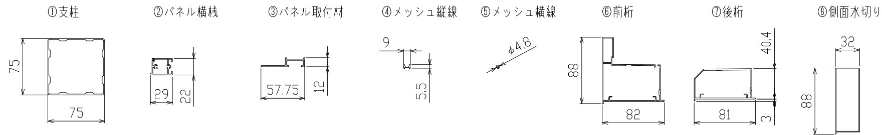
主要部材断面 (S=1/5)
