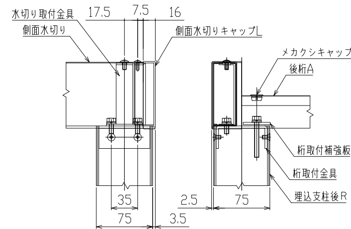
C部詳細図 (S=1/5)
