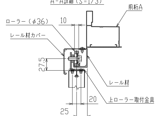
A-A詳細 (S=1/3)
