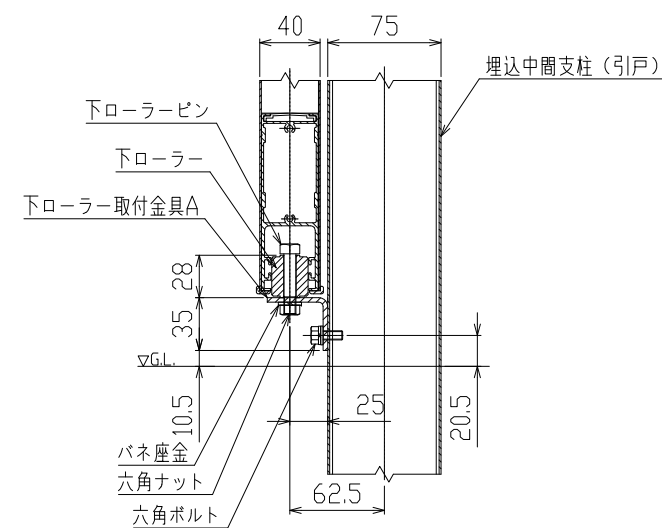
D部詳細図 (S=1/5)
