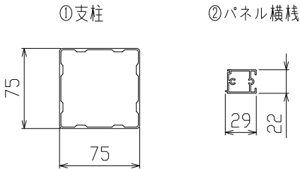
主要部材断面 (S=1/5)
