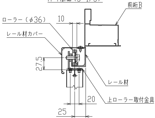
A-A詳細 (S=1/3)
