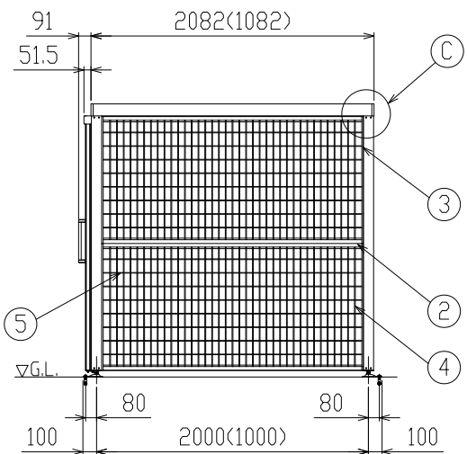
B部詳細図 (S=1/10)
