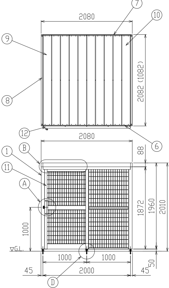
据 付 図 (S=1/50)
