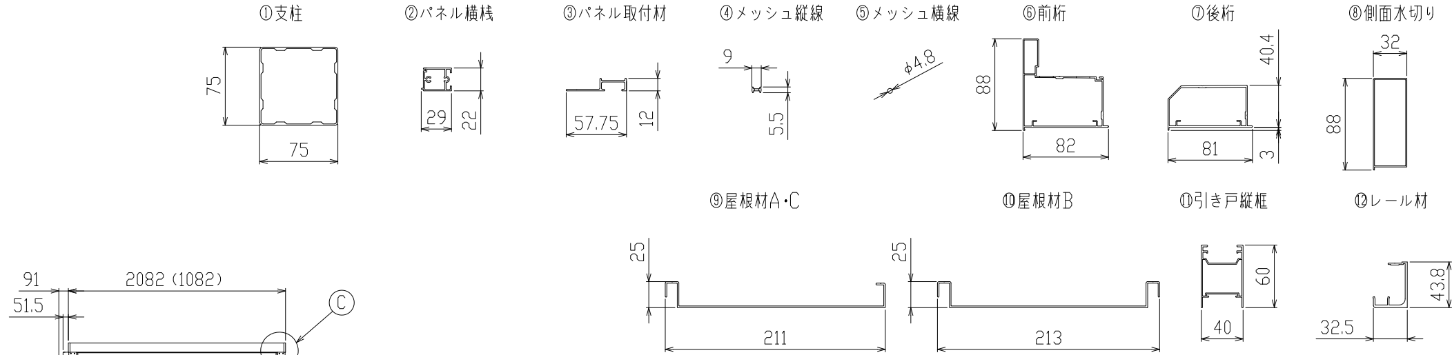
主要部材断面 (S=1/5)
