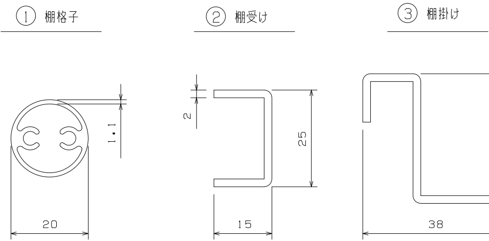
主要部材断面図 S = 1 / 1
