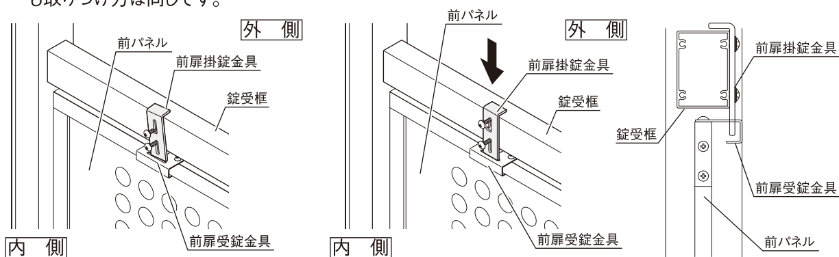
■取付断面図
