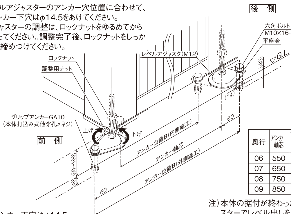
図 13 アンカー施工
