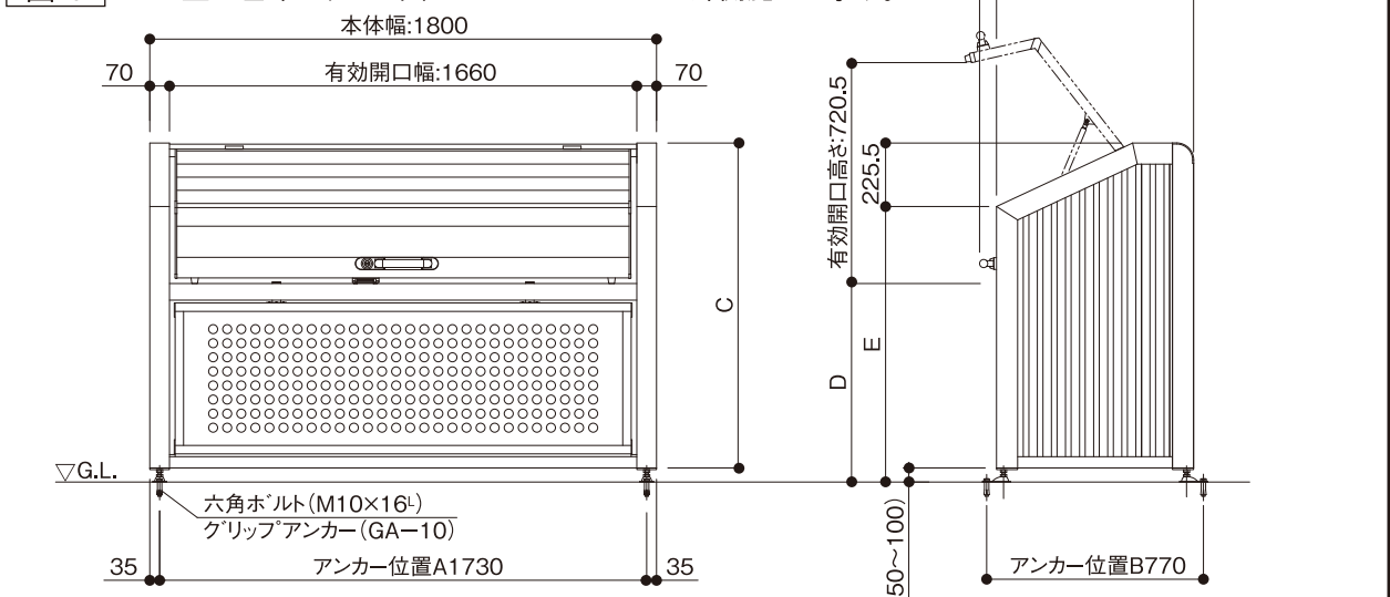
図 2 アンカー設置図(単独) ※図は1812-07アンカー外側施工を示す。
