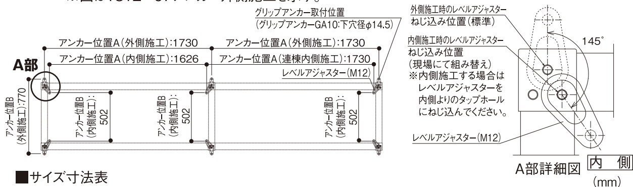
図 12 アンカー設置図(連棟)
