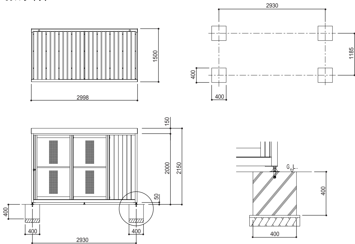
基礎部分拡大図
