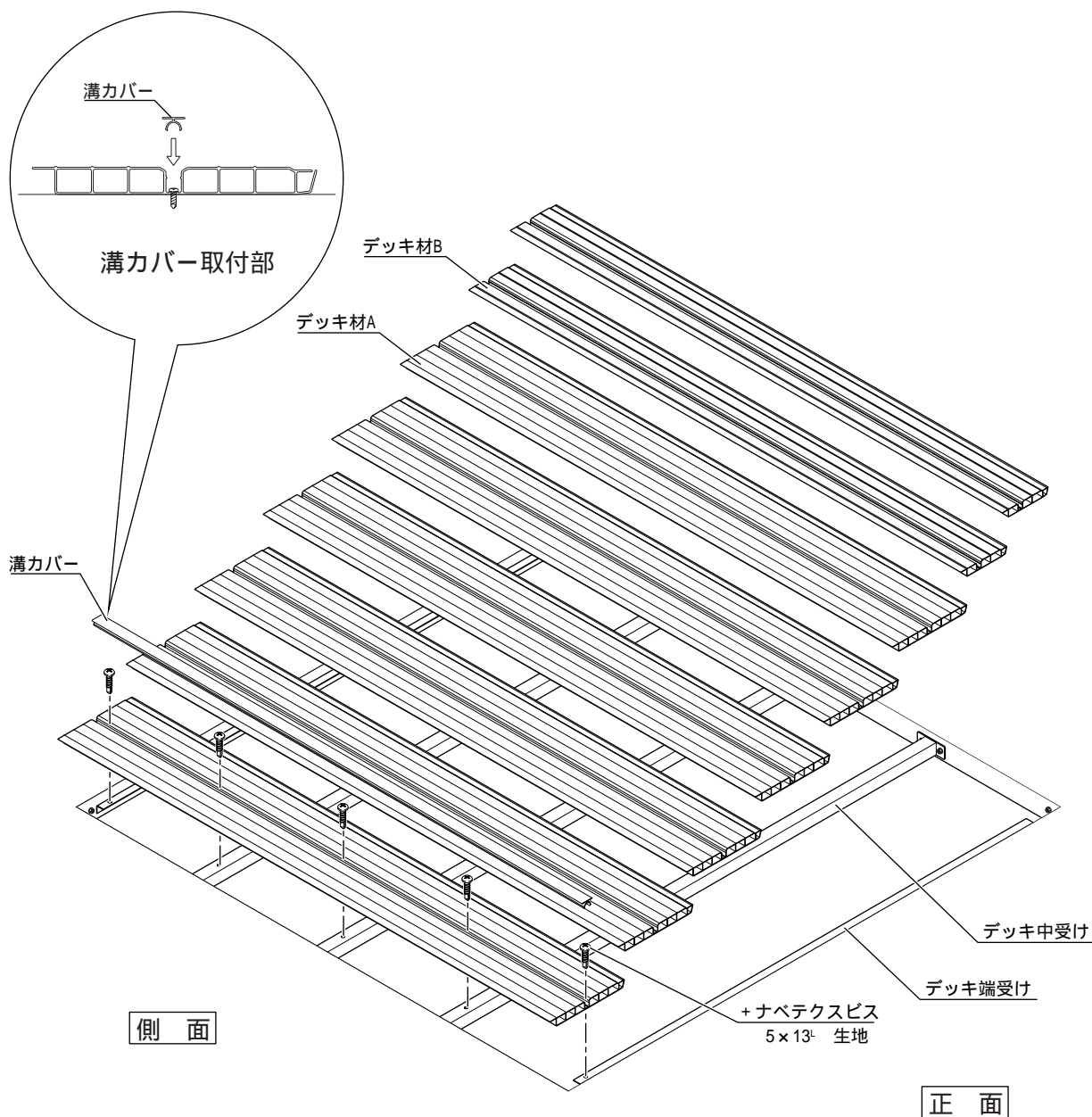
取付部断面
