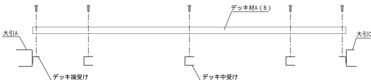
取付部断面
