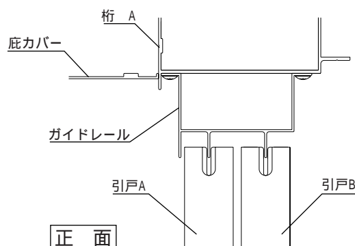
上部取付断面
