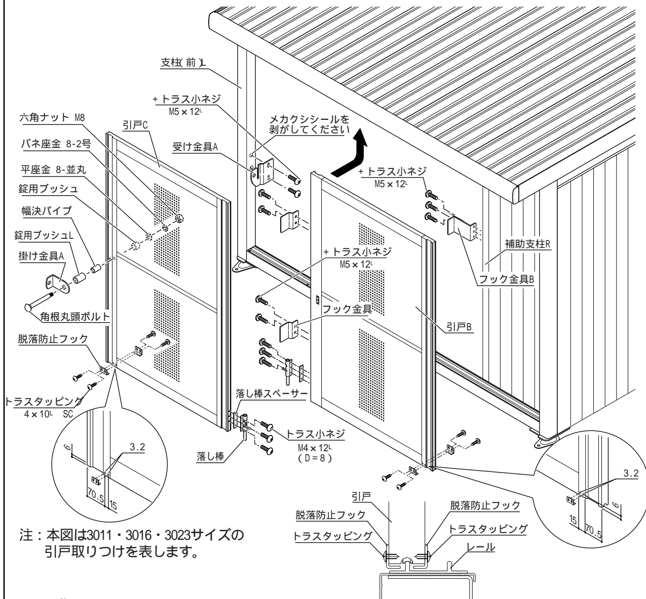
下部取付断面
