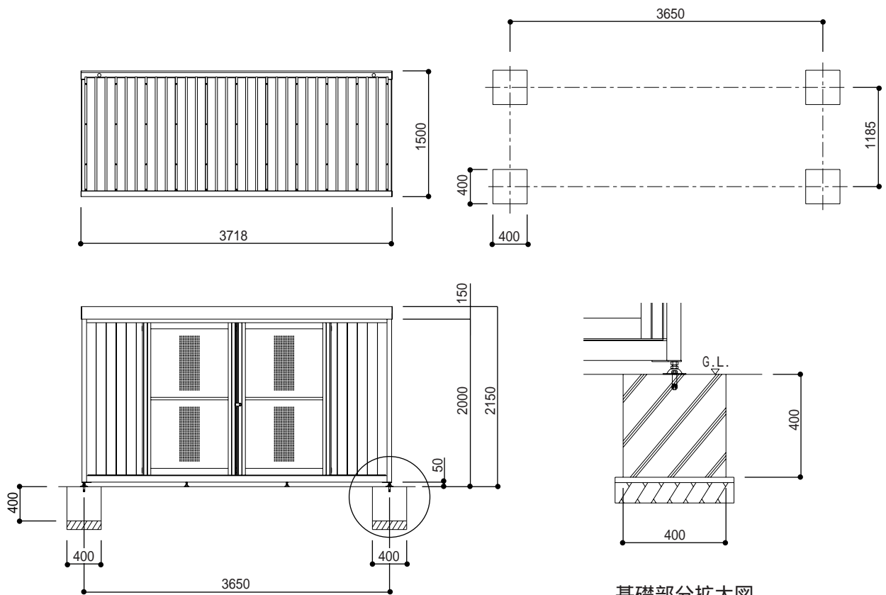
基礎部分拡大図
