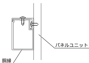
胴縁部断面
