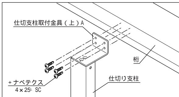
本体中心以外の取りつけ
