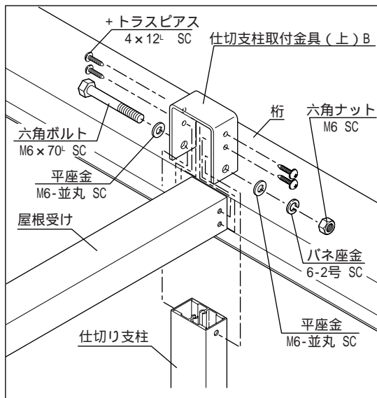
本体中心への取りつけ
