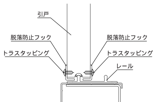
下部取付断面
