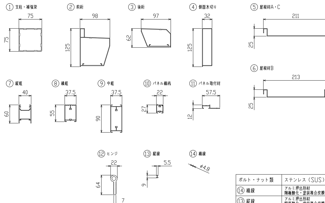
主要部材断面 (S=1/5)
