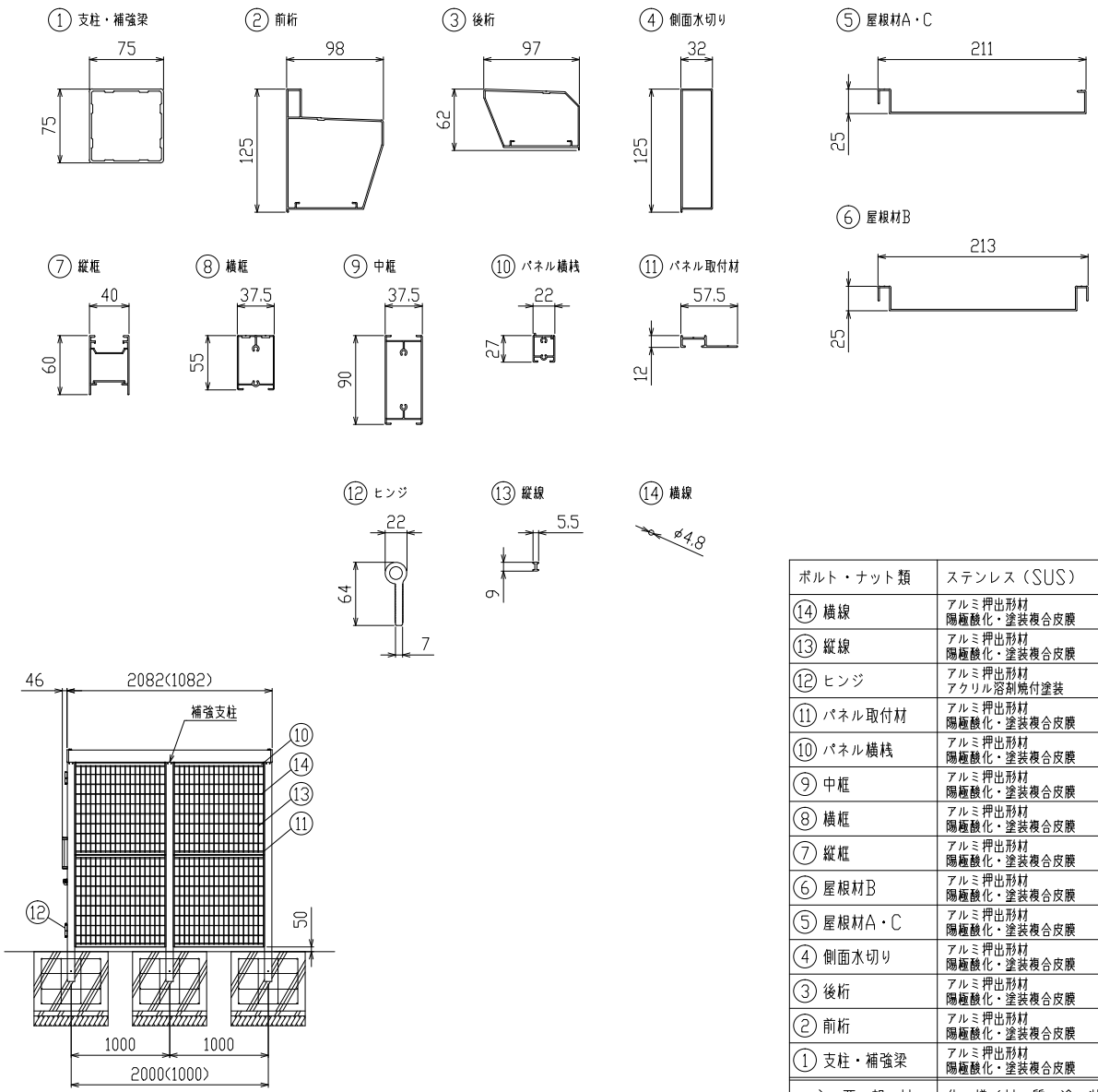
主要部材断面 (S=1/5)
