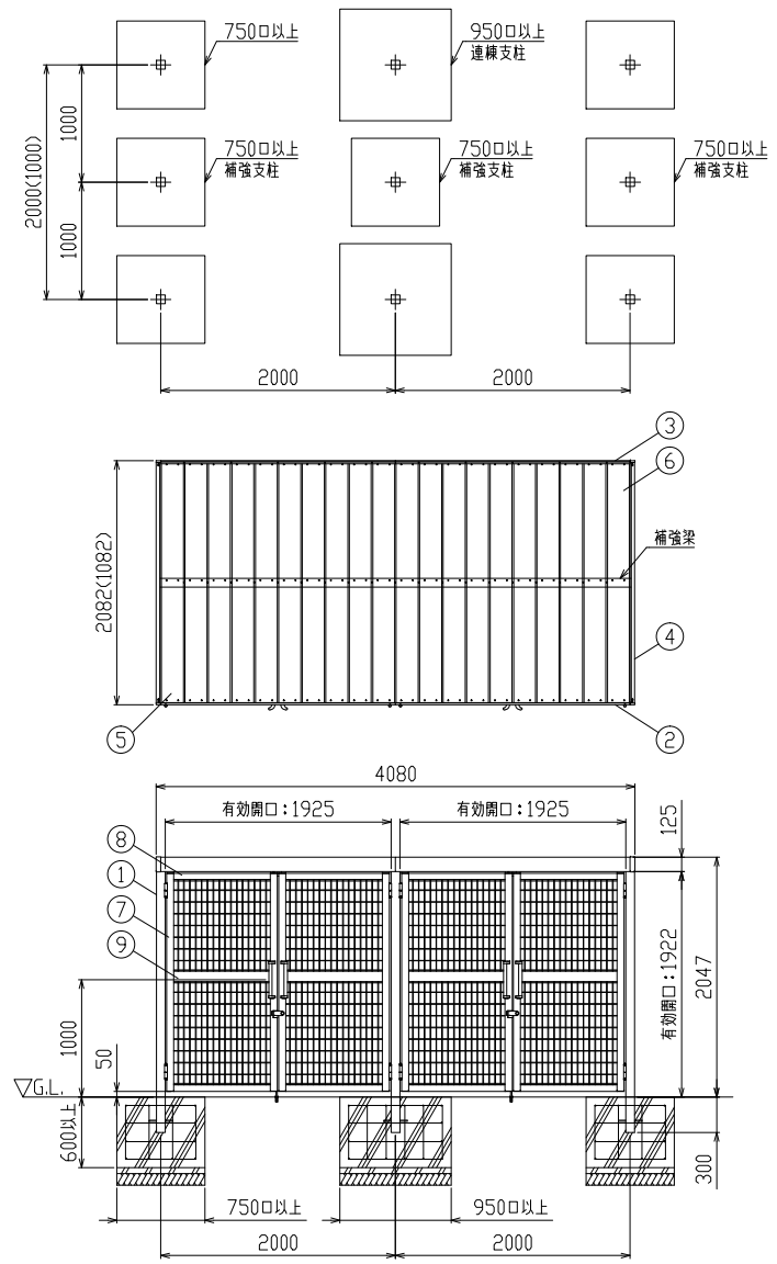
据付図 (S=1/50)
