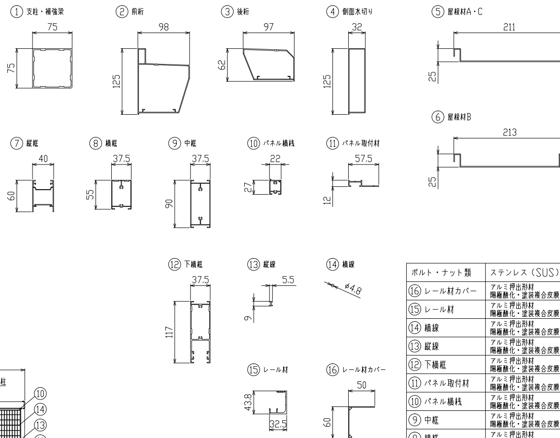
主要部材断面 (S=1/5)
