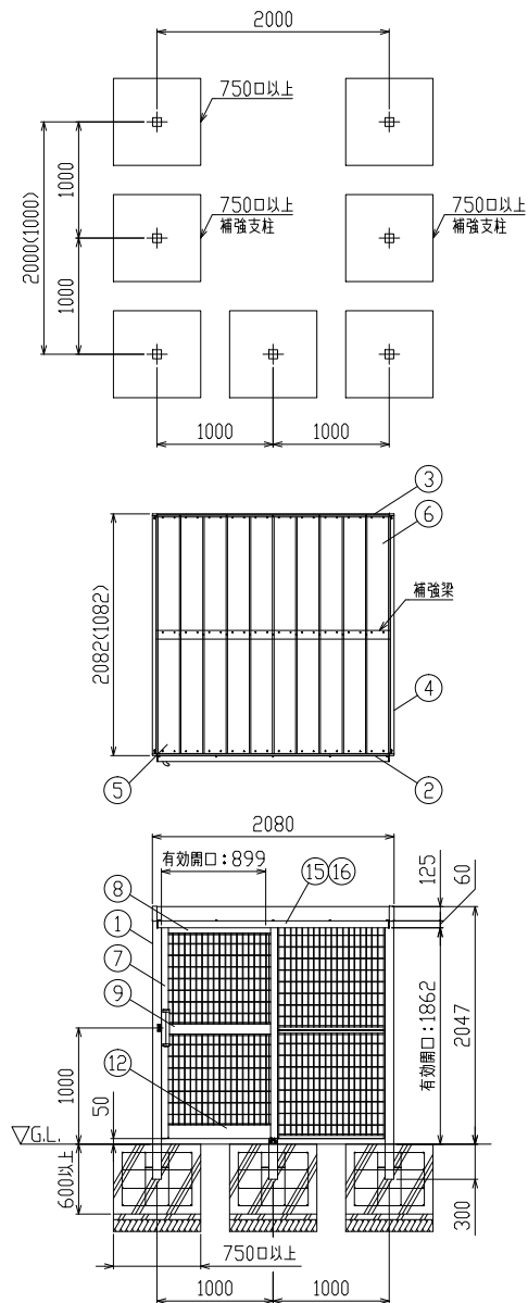
据付図 (S=1/50)
