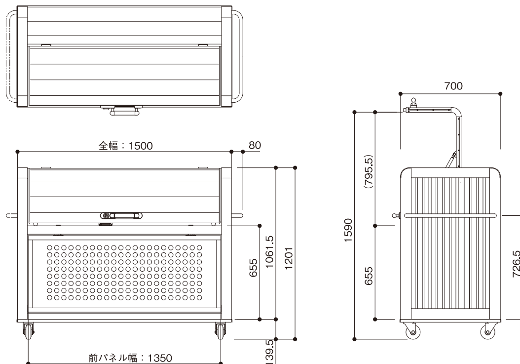
図 1 GPJ型 基本セット (GPJ-1512-07SC)
