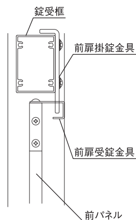
■ 取付断面図
