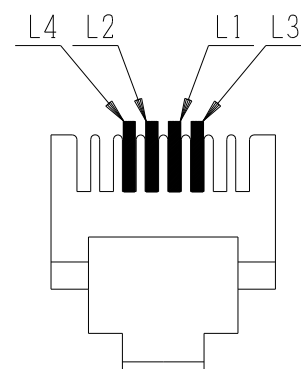
■接触ピンの接続図(正面図)
