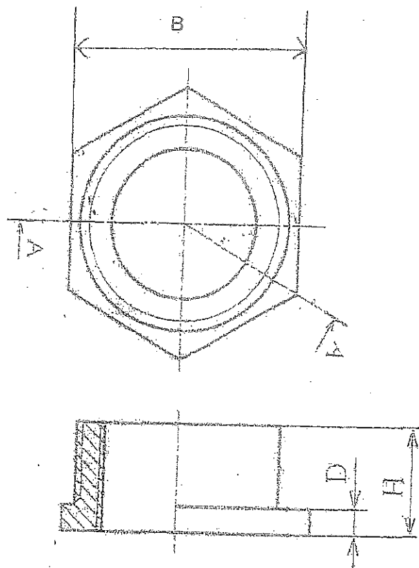
A-A' 断面
