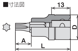
■寸法図
