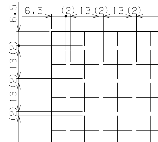
切り込み詳細 (S=1/1)
