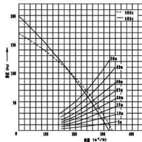
■ 静圧・風量特性 (グリッフィルターDV-182F標準時)
