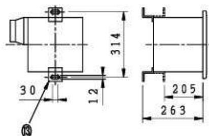
■ 吊下金具取付位置
