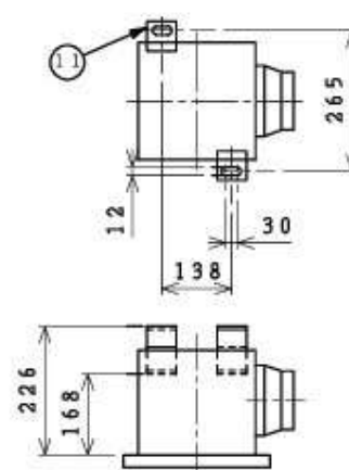
■吊下金具取付位置
