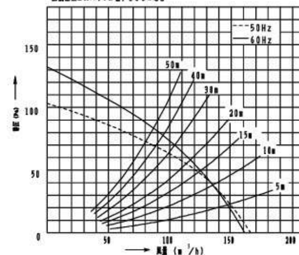
● 測定-風量特性 (ブリスフィルターDVF-142F製品8時)
