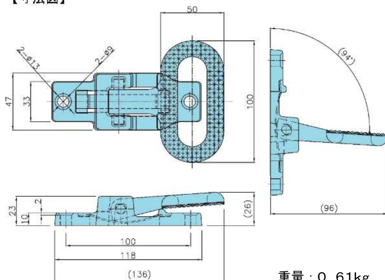
【寸法図】
