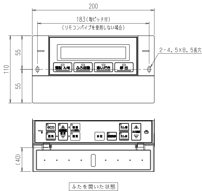
浴室リモコン RC-3321S
