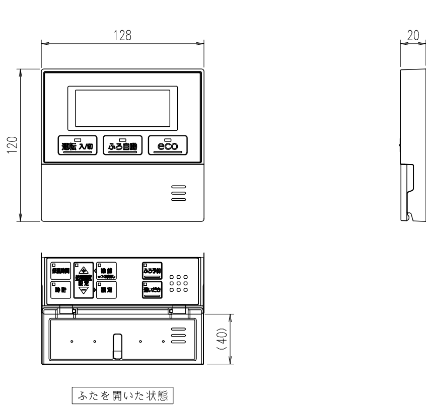
台所リモコン RC-3321M
