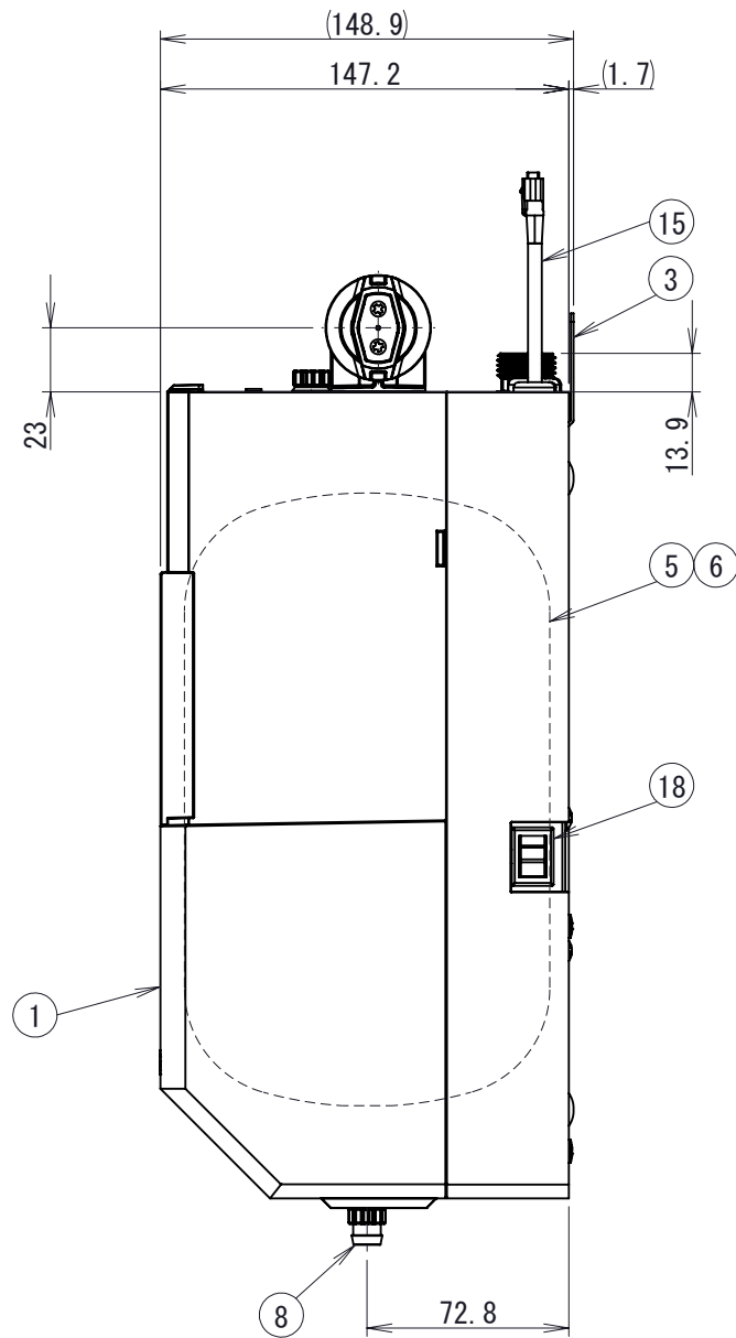
正面カバー取り外し状態詳細図
