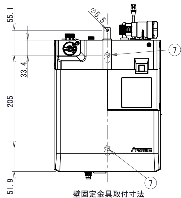
壁固定金具取付寸法
