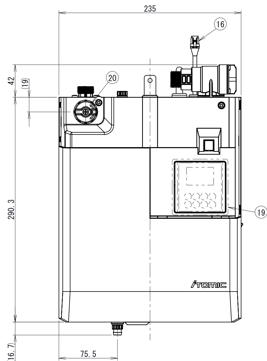
正面カバー取り外し状態詳細図
