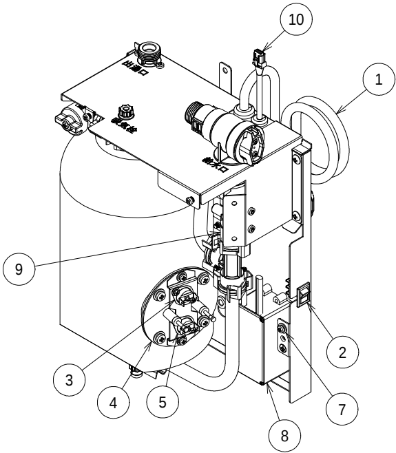
部品配置図 ESWM3ASS
