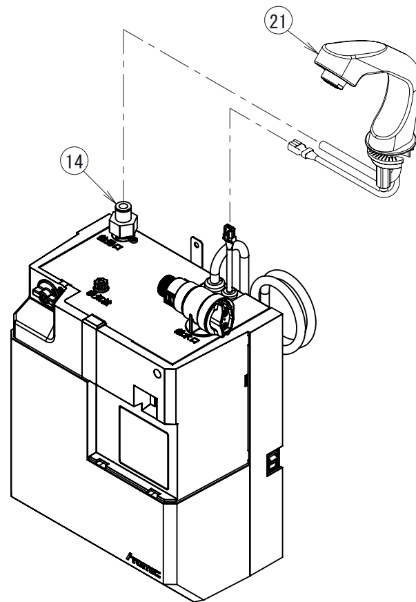
アイソメ図《自動水栓組立》
