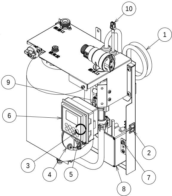
部品配置図 ESWM3TSS
