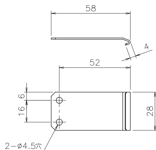
■給気カバー 取付板（S=1／3）
