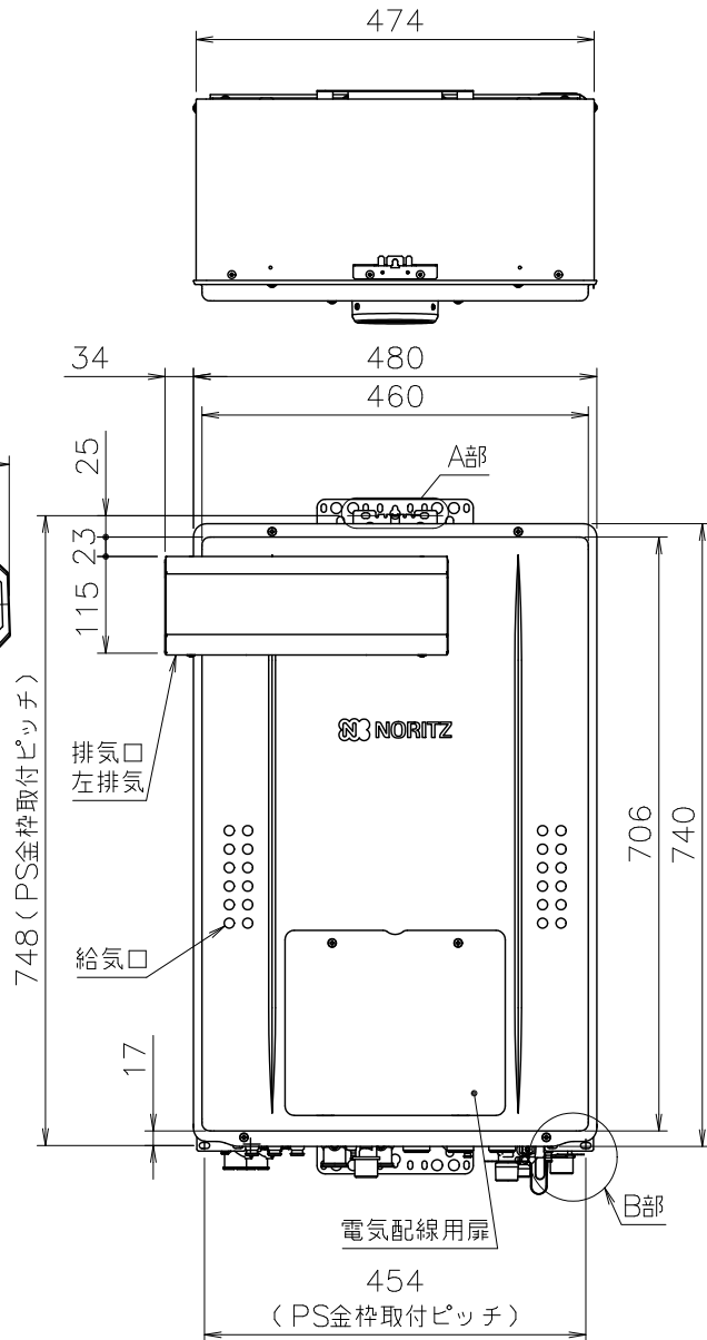
748 (PS金枠取付ピッチ) 100 70 40 2×6.5×10長穴 1.2 12 12 17 85° 10 12 18 170 70 36 6×6×10長穴 壁取付用穴 4×φ13穴 絶縁部品用取付穴 21 10 43 114 100 140 205 R4.5 130 781 721 140 100 6×6×10長穴 壁取付用穴 4×φ13穴 絶縁部品用取付穴 24 41 240 10 36 70 170 7×12.5長穴 23 9 ■ B部詳細図 (尺度1/2) 標準設置形Ⅱ型 (図番W-00-0335) 適応金枠 参考図面
