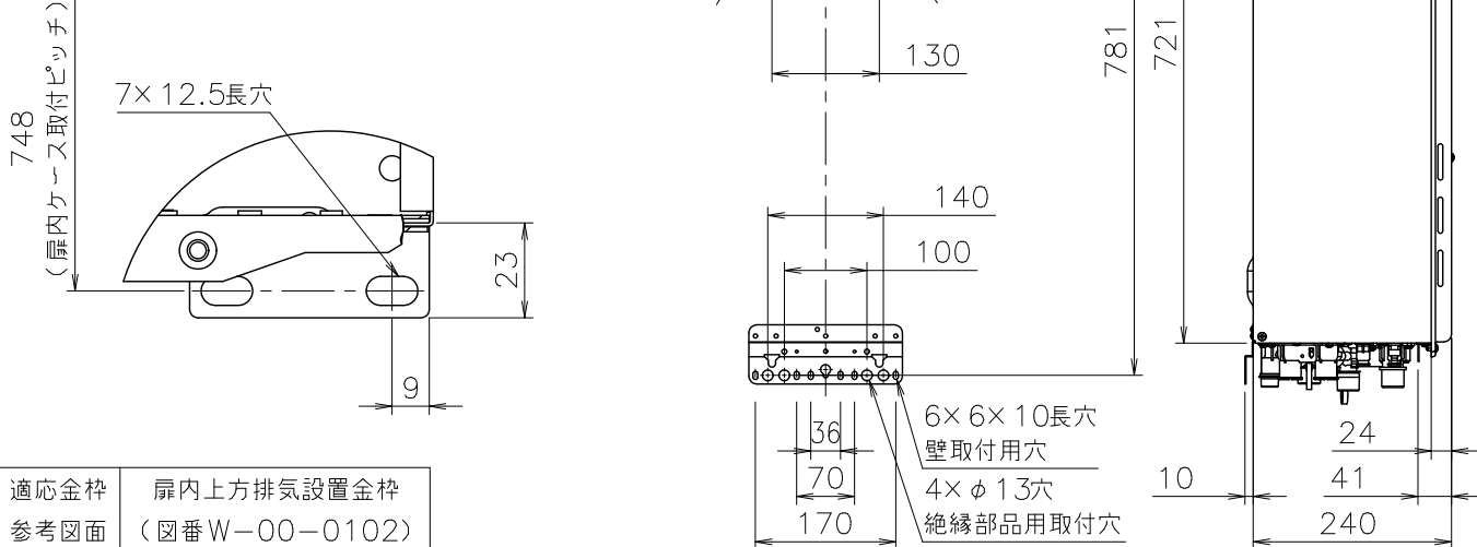
■B部詳細図 (尺度 1/2)
