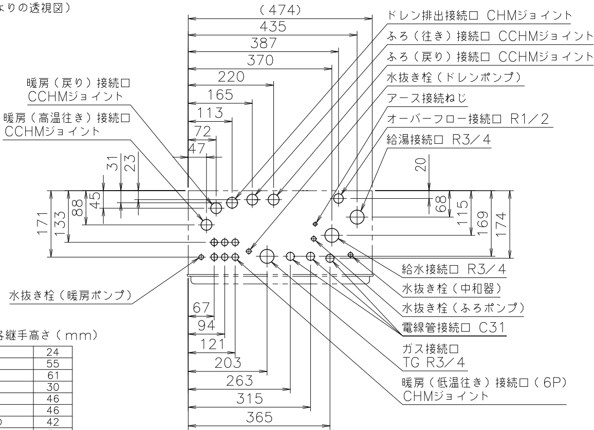
(単位：mm) (機器上方よりの透視図)
