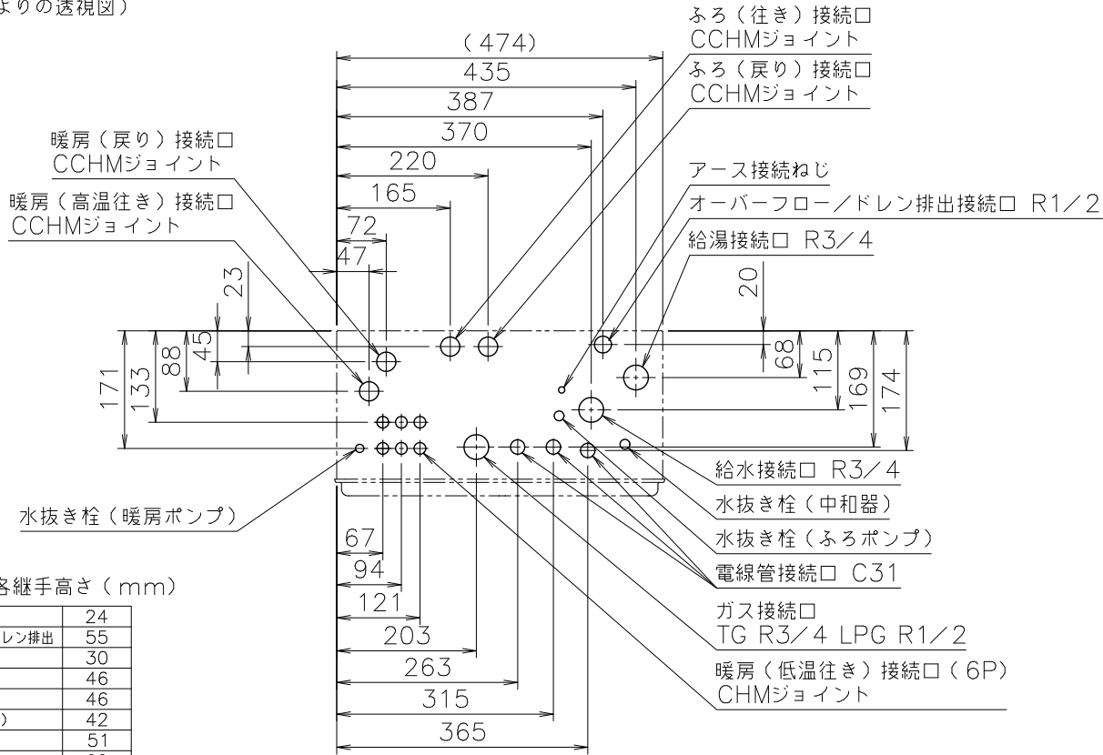
■追いだき配管条件
