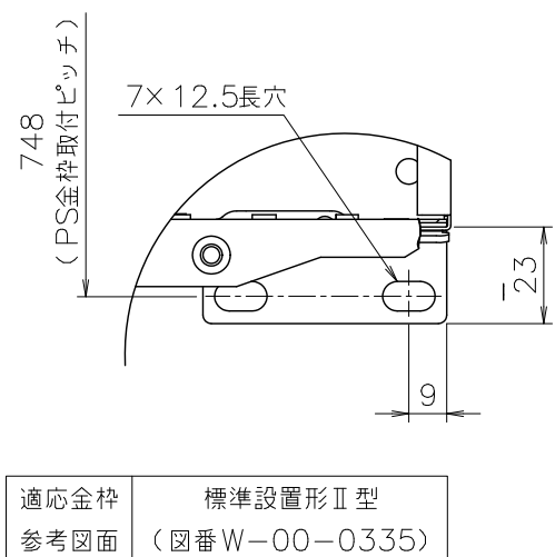
■B部詳細図 (尺度1/2)
