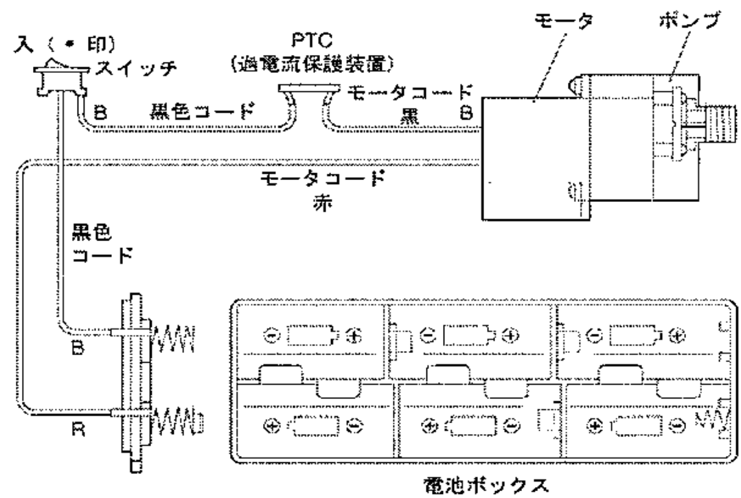
実体配線図
