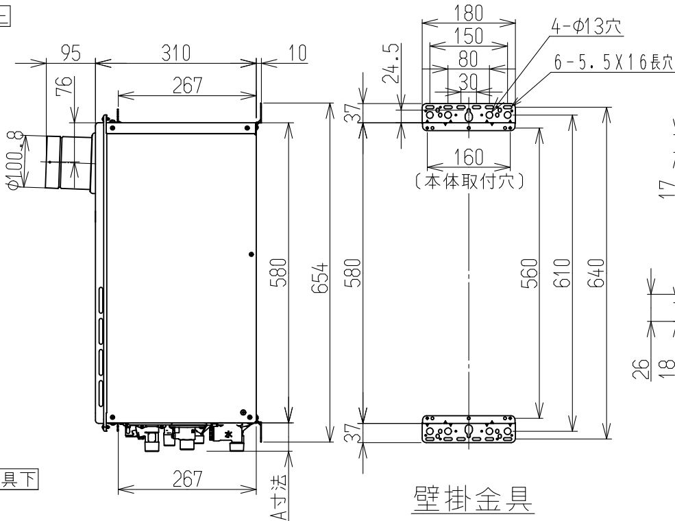
●トリイ配管を行う場合
